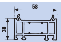
Blendrahmenver- breiterung 3 cm
