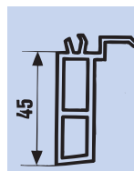
Fensterbankan- schlußprofil 4,5 cm
