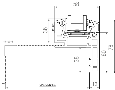
Drawing: Klickfix 58 - FIB
