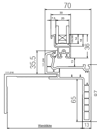
Drawing: Klickfix 70- PLUS
