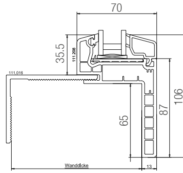
Drawing: Klickfix 70 - FIB
